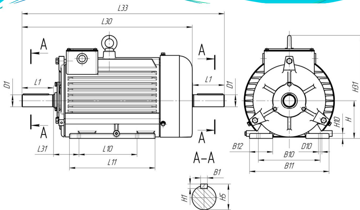
Конструктивное исполнение 4MTKF 132 IM 1001, IM 1002
