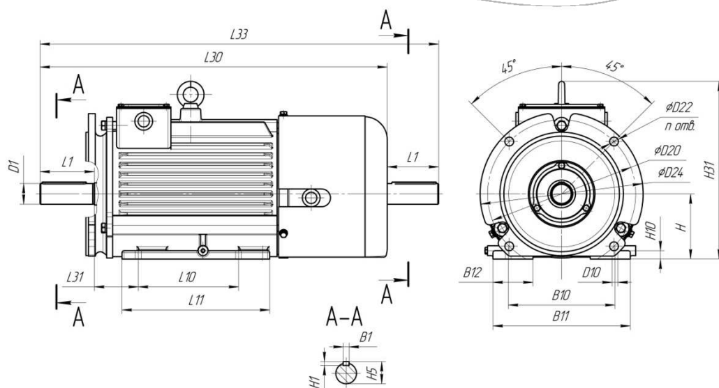
Конструктивное исполнение IM 2001, IM 2002
