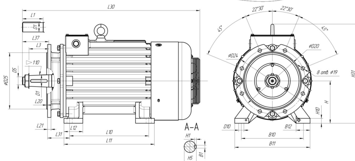
Конструктивное исполнение ИМ 2001, ИМ 2003
